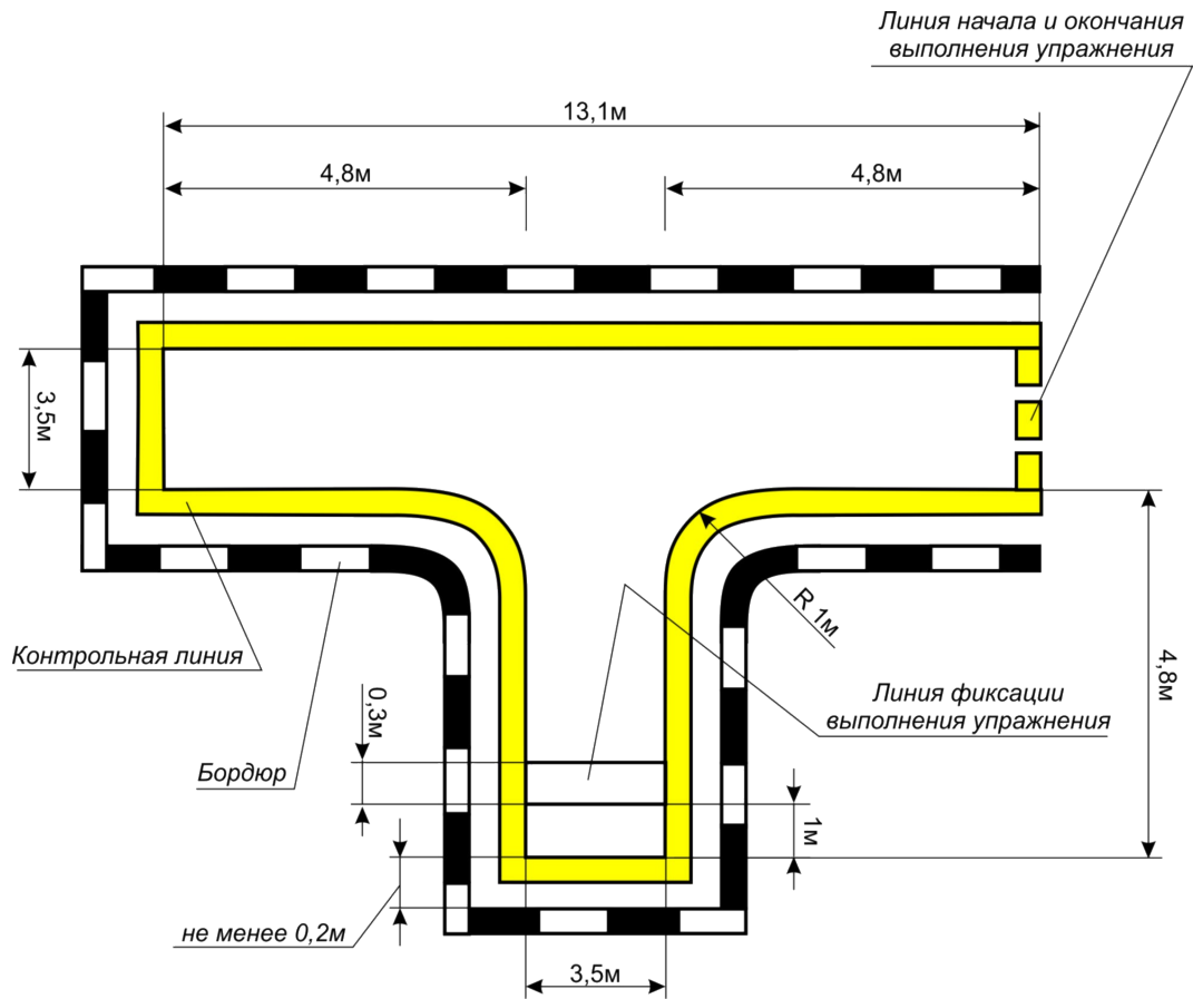
Рис.17. Зона упражнения № 6 «Разворот и парковка» для категории «B»
