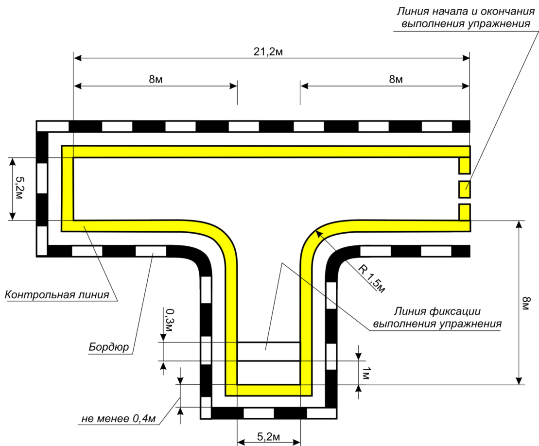
Рис.18. Зона упражнения № 6 «Разворот и парковка» для категорий «C», «D»
